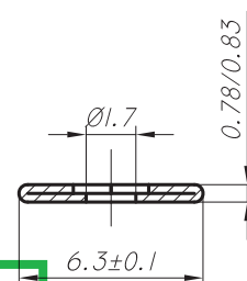
CORTE C-C
